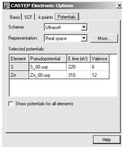
Рис. 3.18. Вкладка задания параметров псевдопотенциала
