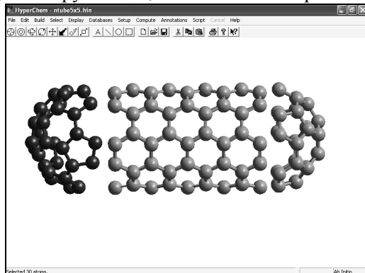
Рис. 2.34. Стыковка второго фрагмента фуллера C_{60} с нанотрубкой
