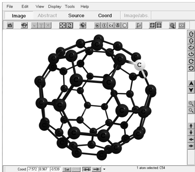
Рис. 1.1. Поле визуализации программы ChemCraft. Расчет оптимизированной конфигурации структуры фуллера C 60 с помощью программы Gamess
